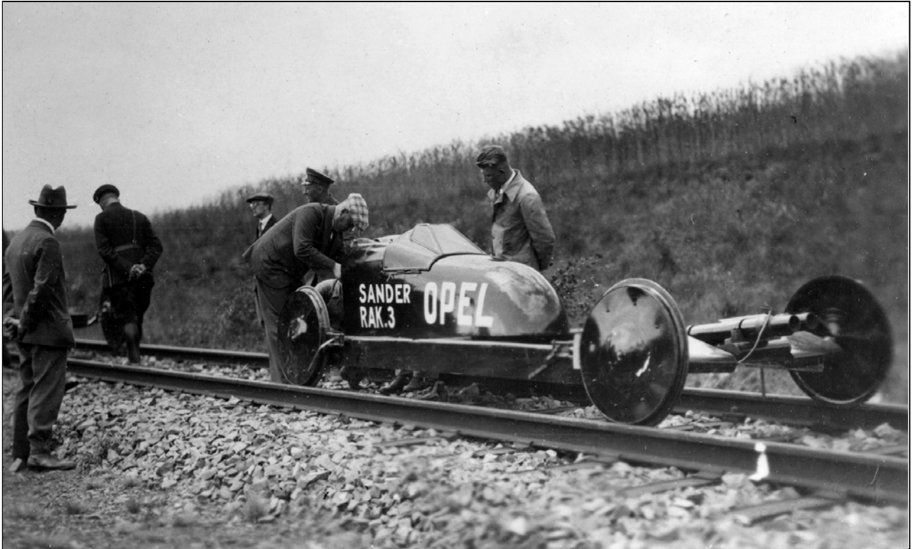
Fritz von Opel und Ingenieur Friedrich Wilhelm Sander am 23. Juni 1928 am Raketen-Schienefahrzeug RAK 3. Foto: Opel Classic Archiv
